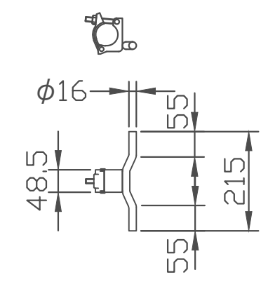
丁番クランプ詳細
